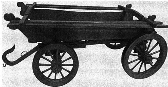
Boerenwagen | 1e werkstuk gemaakt tussen 15 februari en 28 maart 1977 | Schaal 1 : 10
